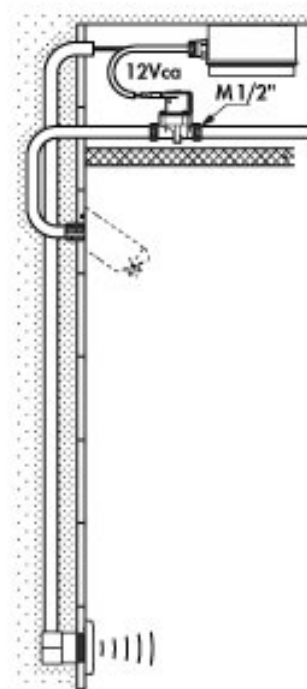
Tempomatic brusesystem med Delabie Round brusehoved
